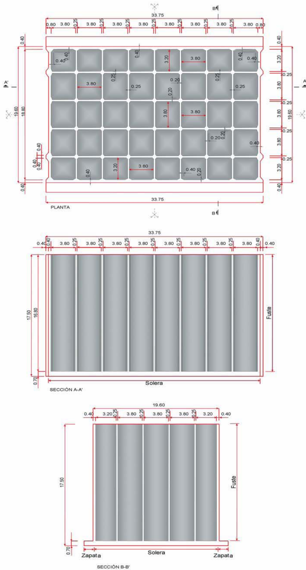
Fig.1 Geometría típica de un cajón flotante
